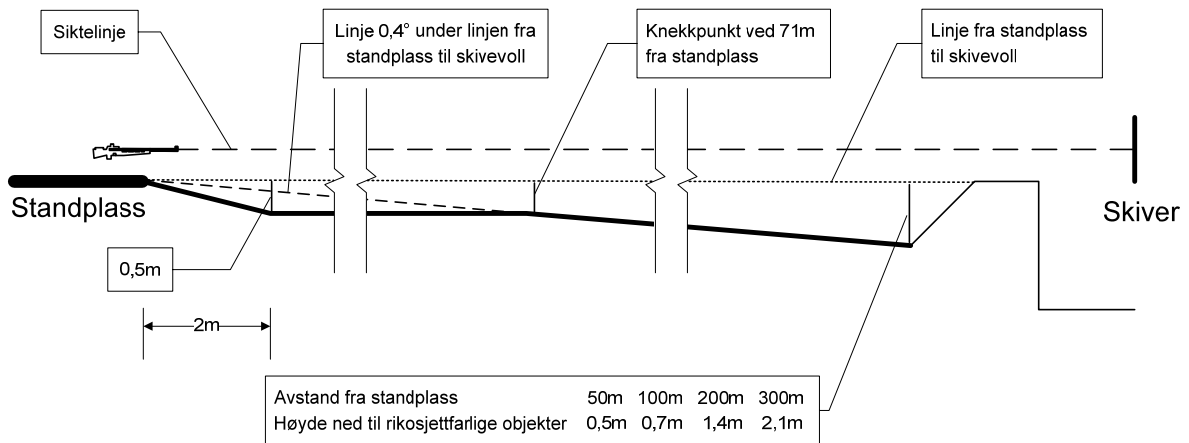
Figur 2 Sektor uten rikosjettfarlige objekter
